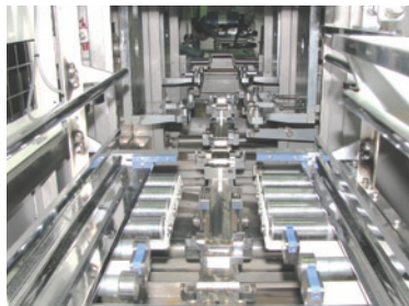
搬入部
